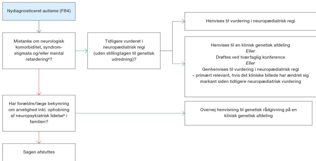
FIGUR 1 Henvisningsalgoritme.
